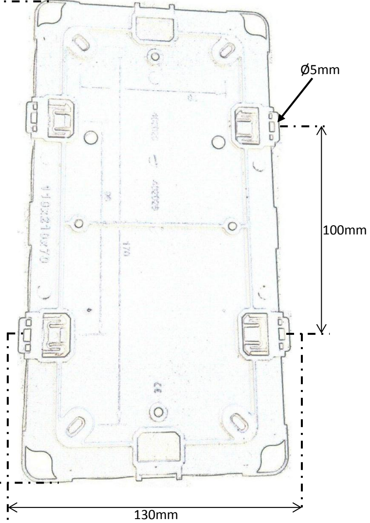
ALTAN GÖRÜNÜŞ /BOTTOM VIEW
